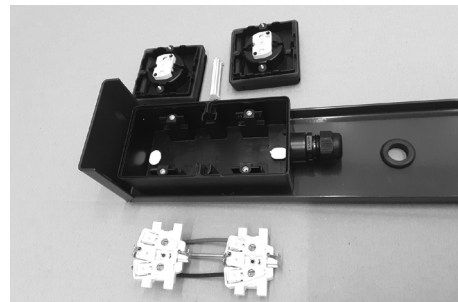
Stap 3. Verwijder de witte contactdelen door tussen het witte gedeelte en de vergrendel-nokken met een platte schroevendraaier voorzichtig te wrikken zodat één zijde van de witte contactdelen los komt. Verwijder het contactgedeelte uit de vergrendel-nokken.
