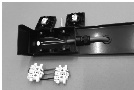
Stap 4. Buitenkabel Wees er van overtuigd dat er geen spanning op de kabel staat. Strip een geschikte kabel en manoeuvreer deze via de opening in de tuinpaal (ter bescherming van de kabel is een rubber ring toegepast) door de wartel naar de binnenzijde van de onderbak.
