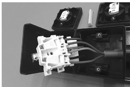
Stap 5. Wees er van overtuigd dat er geen spanning op de kabel staat. Steek de gestripte aders, bij de voorbedraaide contacten, in het witte contactgedeelte. Houdt onderstaande volgorde aan: Blauw bij blauw = N (nul), Geel/groen bij geel/groen = aarde. Zwart bij bruin = L (fase).
