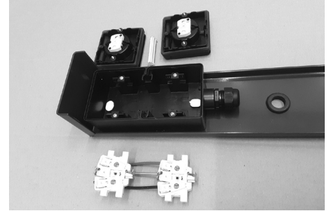
Stap 3. Verwijder de witte contactdelen door tussen het witte gedeelte en de vergrendel-nokken met een platte schroevendraaier voorzichtig te wrikken zodat één zijde van de witte contactdelen los komt. Verwijder het contactgedeelte uit de vergrendel-nokken.
