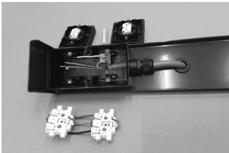
Stap 4. Grondkabel Wees er van overtuigd dat er geen spanning op de kabel staat. Strip een geschikte (grond)kabel en manoeuvreer deze via de opening in de tuinpaal (ter bescherming van de kabel is een rubber ring toegepast) door de wartel naar de binnenzijde van de onderbak.
