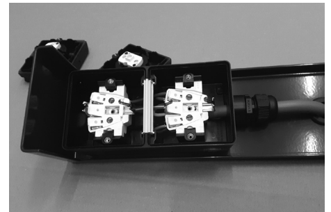
Stap 6. Druk de witte contactdelen weer terug op hun plaats in de onderbak en vergeet niet het "tussenschotje" terug te plaatsen.
