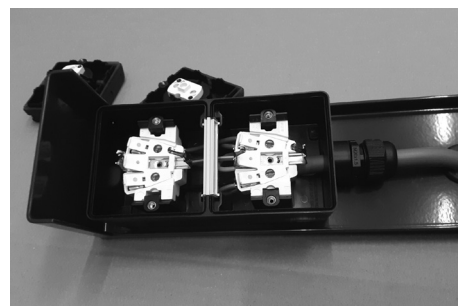
Stap 6. Druk de witte contactdelen weer terug op hun plaats in de onderbak en vergeet niet het "tussenschotje" terug te plaatsen.
