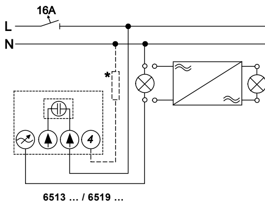
Afb. 4: Dimmerbedrijf met spanningssensor
