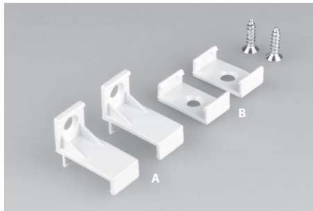
Bevestigingsbeugels.
