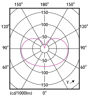
LEDcandle MAS B35 3,4W E14 927 FR-LDD
