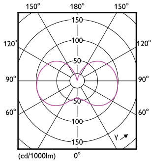
LEDbulb MAS SLR G93 5,9W E27 927 CL-LDD
